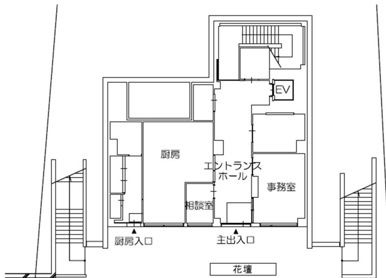
【1階平面図】
